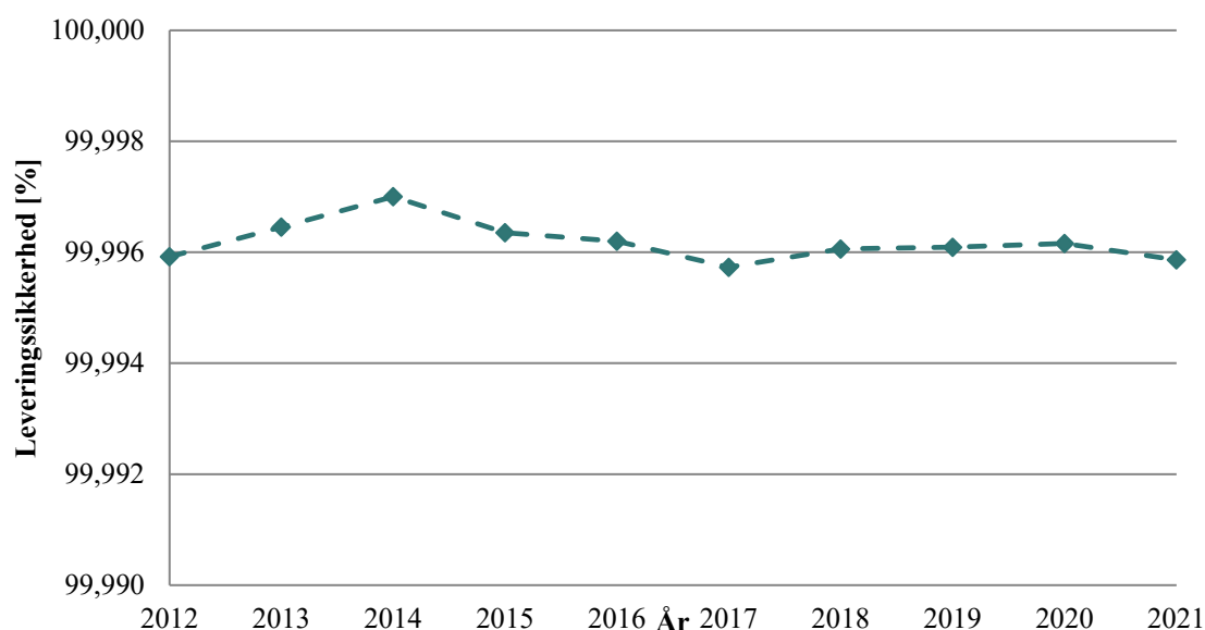
Figur 4.1 Leveringssikkerhed i procent pr. år, ASAI 6
