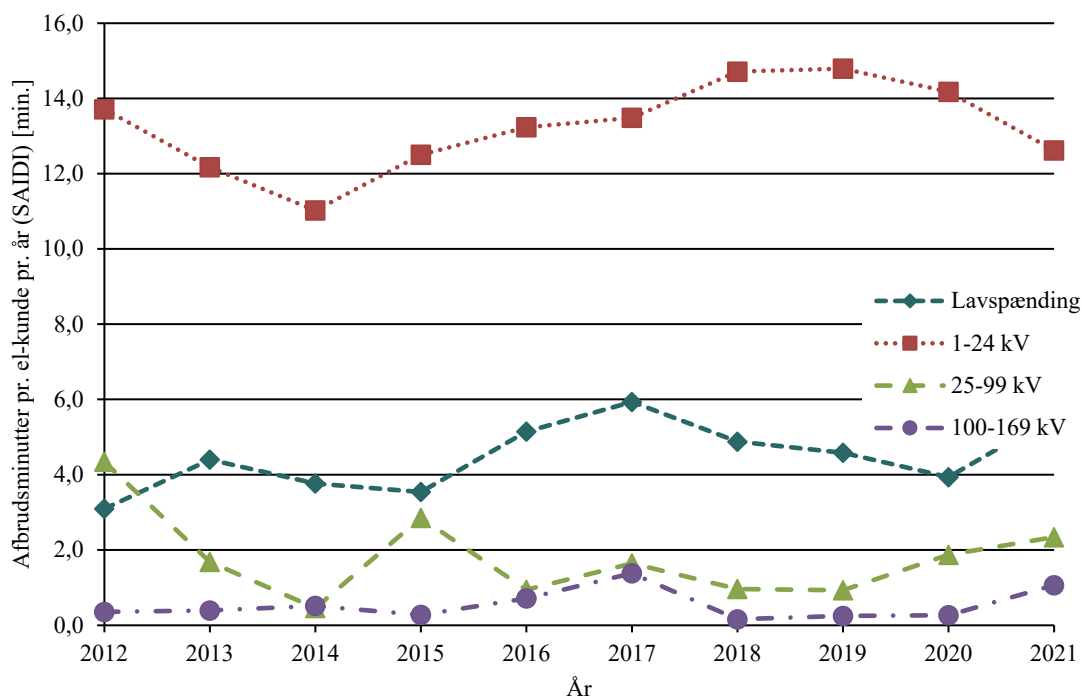
Figur 4.3 Gennemsnitlig afbrudsvarighed pr. kunde i minutter (SAIDI) opgjort pr. udvalgte statistikområder (lavspænding, 1-24 kV, 25-99 kV og 100-169 kV) fordelt på år
