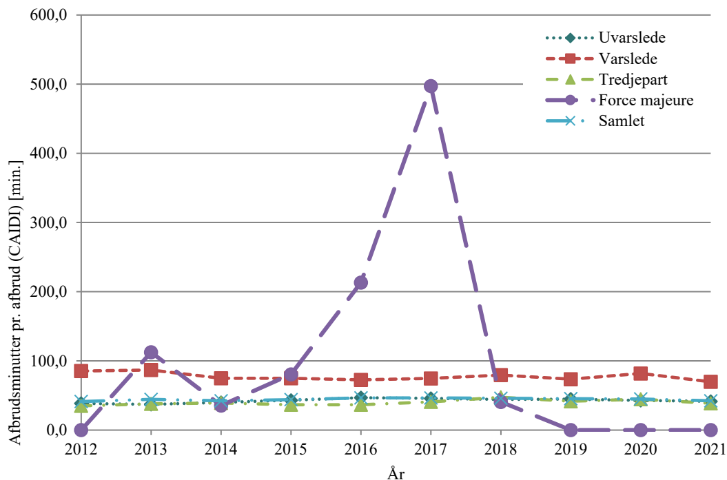
Figur 5.5 Gennemsnitligt antal minutter en kunde er afbrudt ved forskellige typer afbrud (CAIDI)
