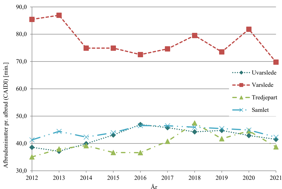
Figur 5.6 Gennemsnitligt antal minutter en kunde er afbrudt ved varslet, uvarslet og tredjepart (CAIDI)
