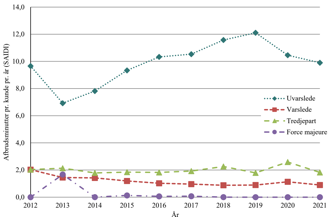
Figur 5.2 Gennemsnitlig kundefbrudsvarighed i minutter opgjort på 1-24-kV-statistikområdet (SAIDI)
