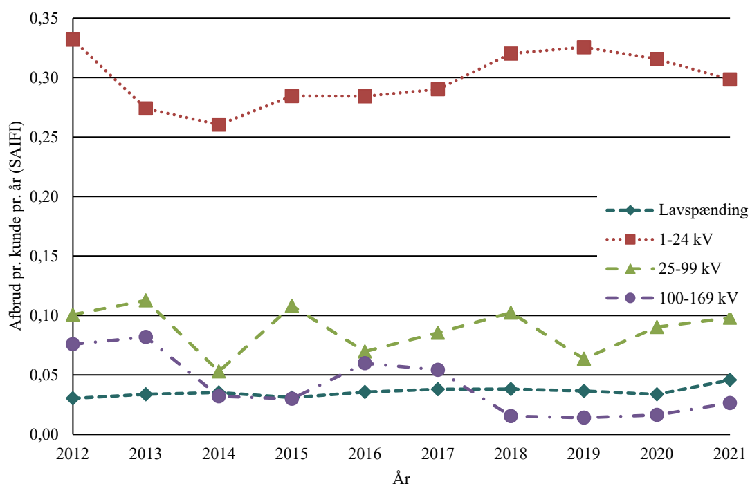
Figur 4.5 Gennemsnitlig afbrudshyppighed pr. kunde opgjort på statistikområderne (SAIFI)
