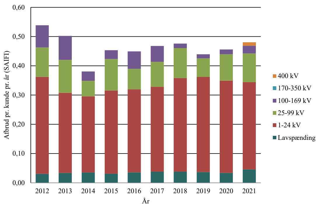
Figur 4.4 Gennemsnitlig afbrudshyppighed pr. kunde opgjort på årstal (SAIFI)
