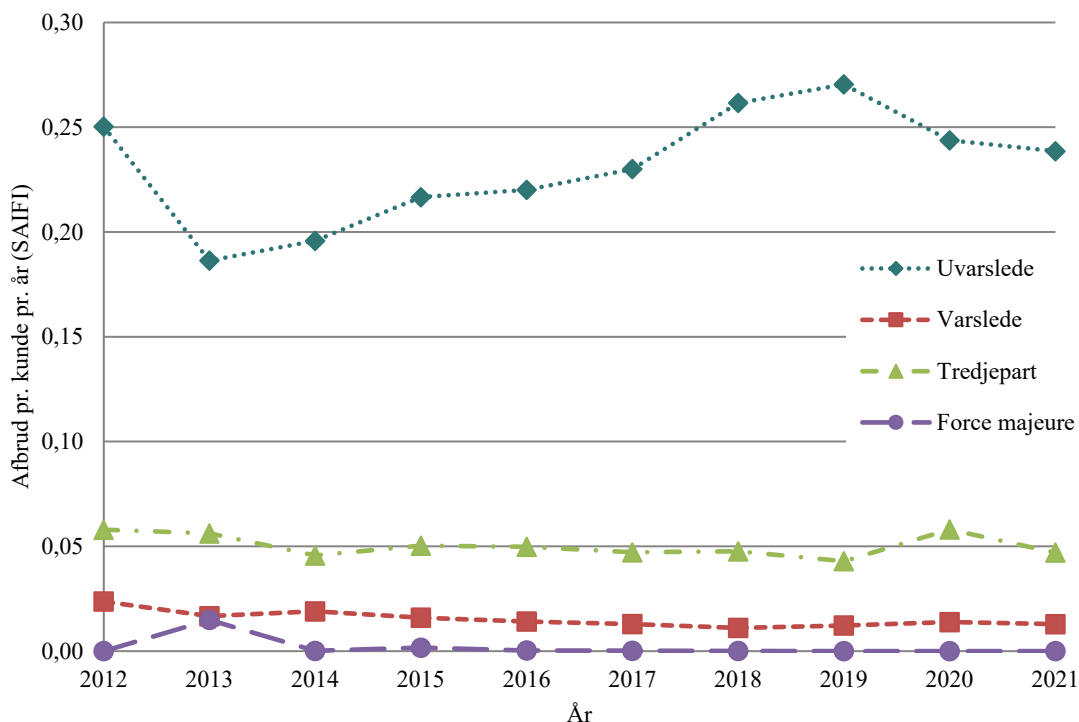
Figur 5.4 Gennemsnitlig kundeafbrudshyppighed opgjort på 1-24-kV-statistikområdet (SAIFI)
