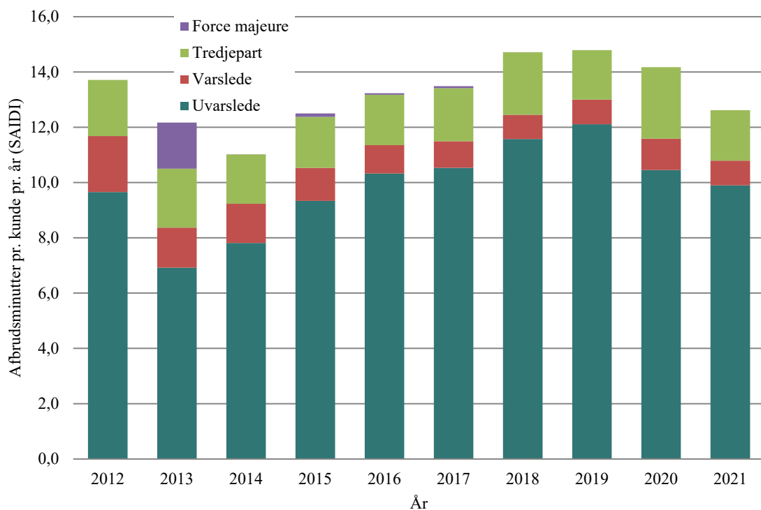
Figur 5.1 Fordelingen af den gennemsnitlige kundeforfbrudsvarighed i minutter opgjort på 1-24 kV-statistikområdet (SAIDI)
