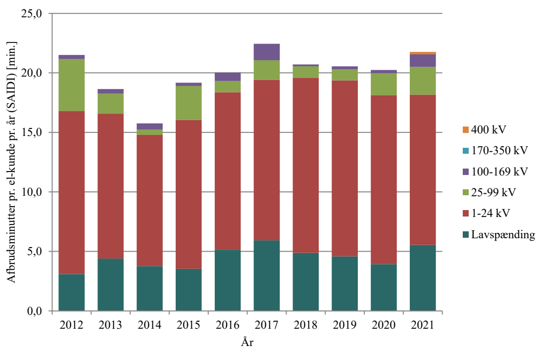
Figur 4.2 Gennemsnitlig afbrudsvarighed pr. kunde i minutter opgjort på statistikområder pr. år (SAIDI)
