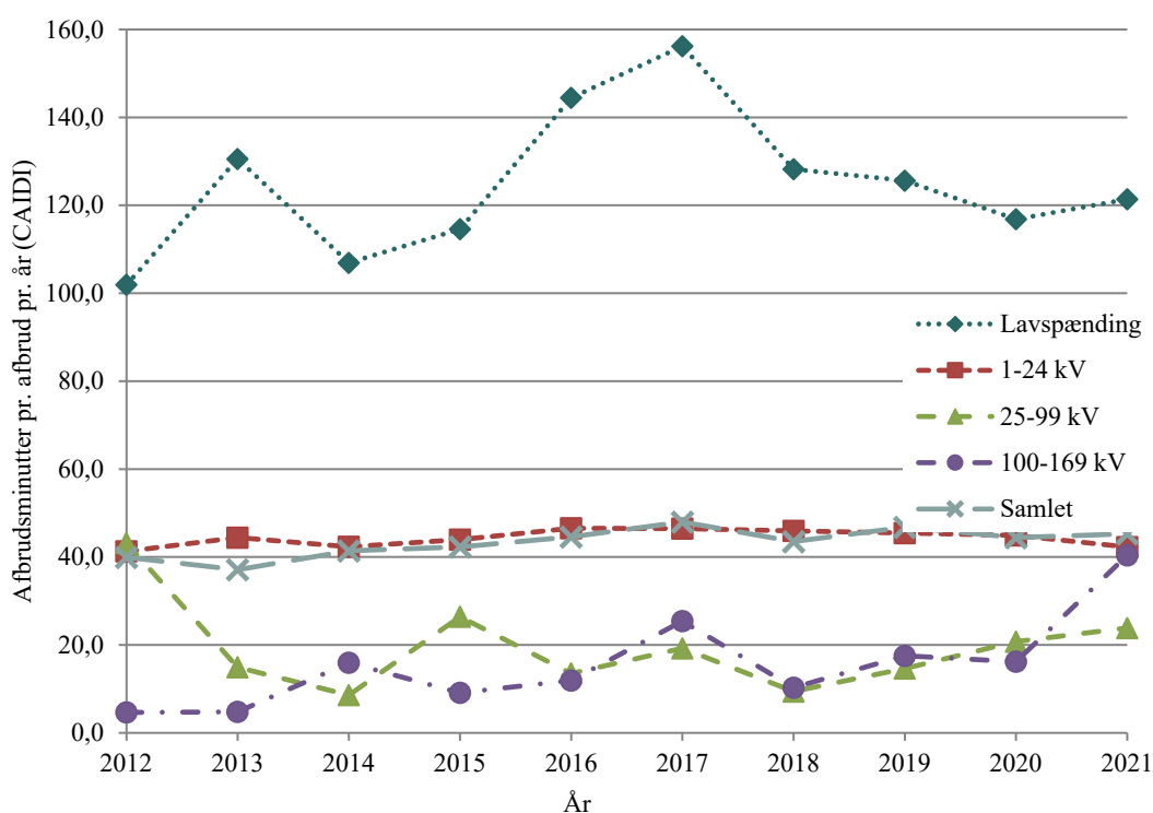
Figur 4.6 Gennemsnitligt antal minutter en kunde er afbrudt opgjort på forskellige statistikområder
